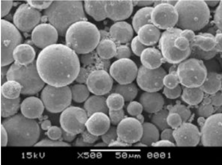
SEM – Cadmium Powder
