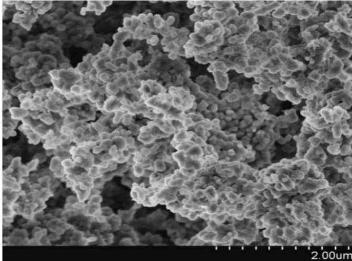
SEM – CaO Powder
