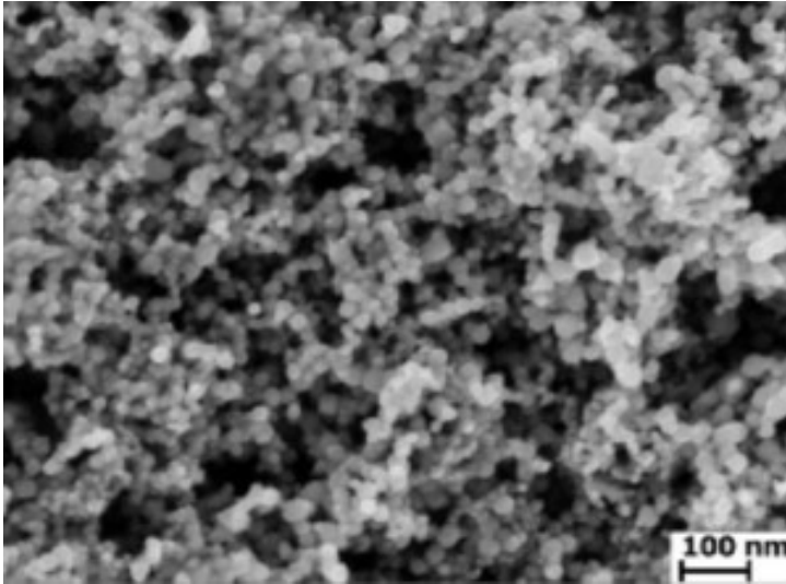
SEM – TiN Powder
