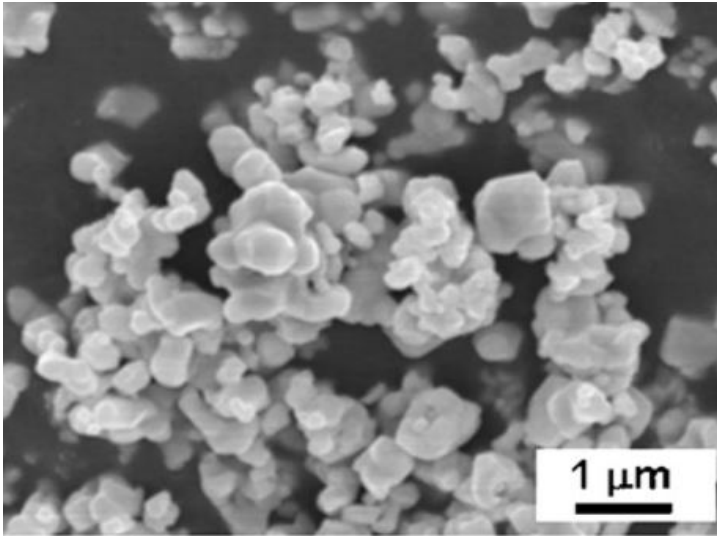
SEM -TaC Powder
