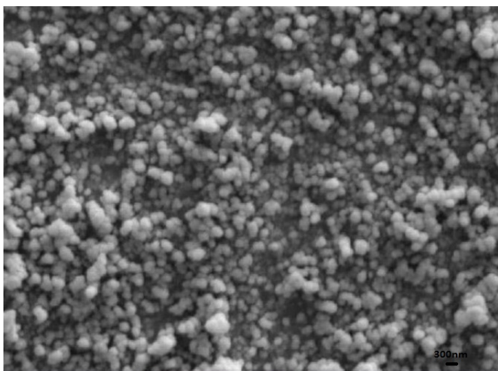
SEM – SrCO 3 Nanopowder
