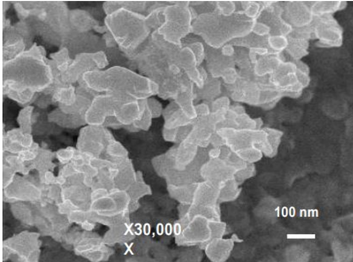
SEM – Tungsten Carbide Cobalt Nanopowder
