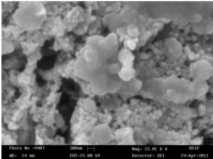
SEM – ATO Nanopowder
