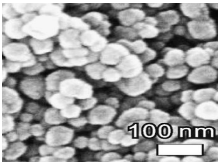
SEM – BaTiO 3 Nanopowder
