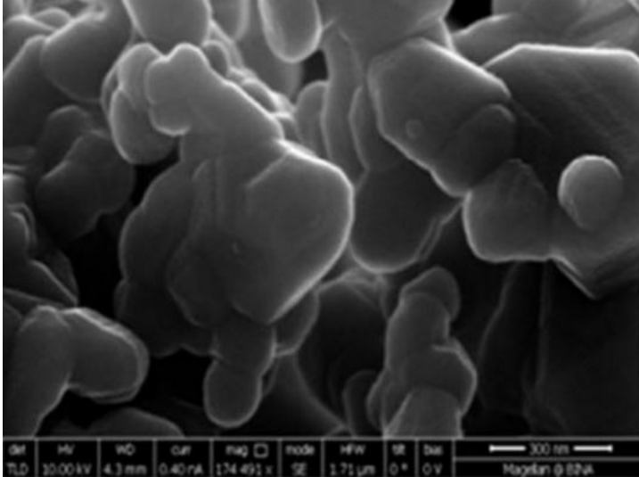
SEM – Strontium Dodecairon Nonadecaoxide
