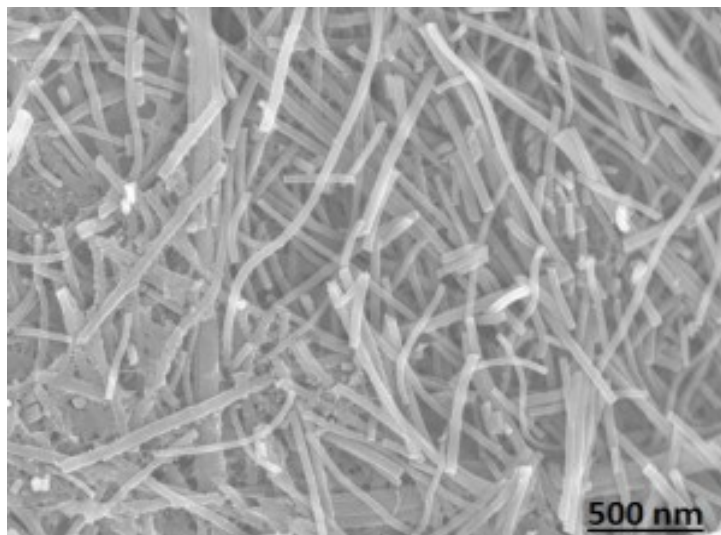
SEM - Carbon NanoFiber
