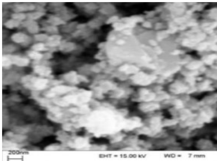
SEM - La 2 O 3 Nanoparticles
