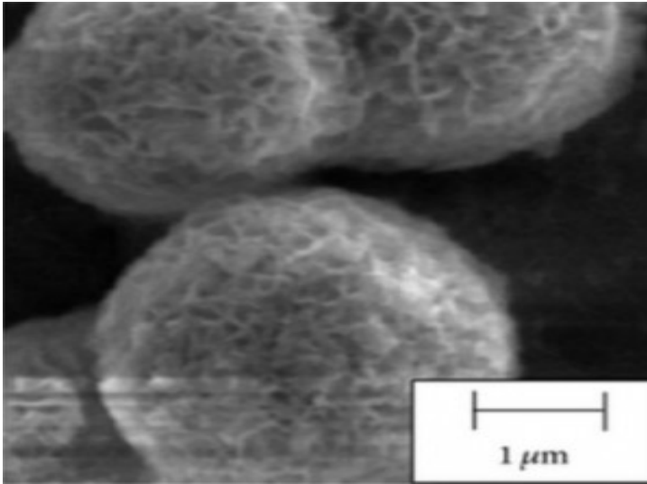
SEM - Fine Cobalt Powder
