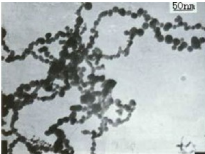
TEM - Nano Iron Powder
