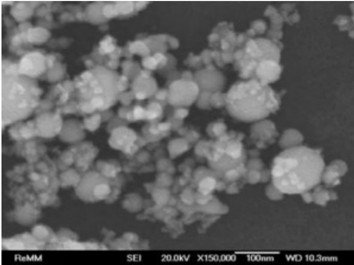
SEM - Tungsten Nanoparticles
