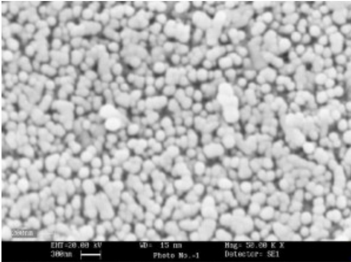
SEM - Zn Nanopowder
