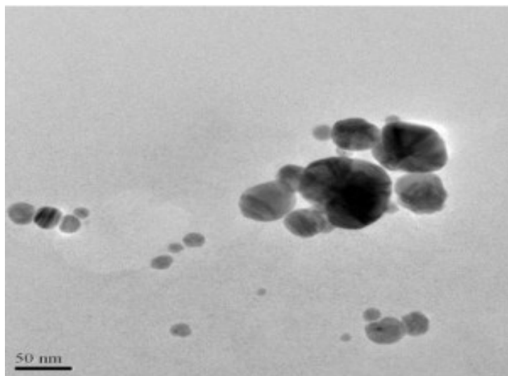
TEM - Manganese Nanopowder
