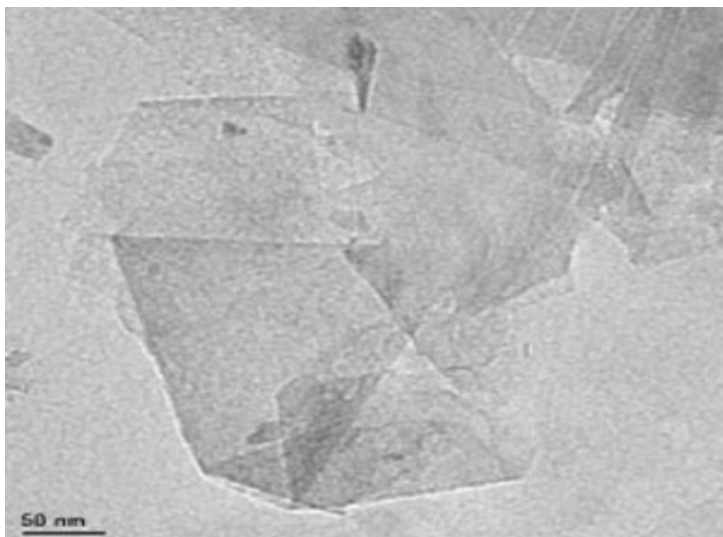
TEM - Graphite Nanoplatelets
