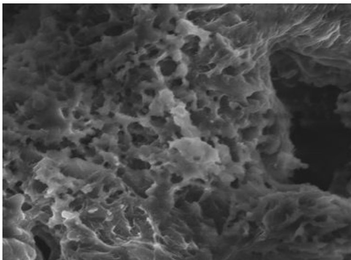
SEM - LiBH 4 Nanopowder
