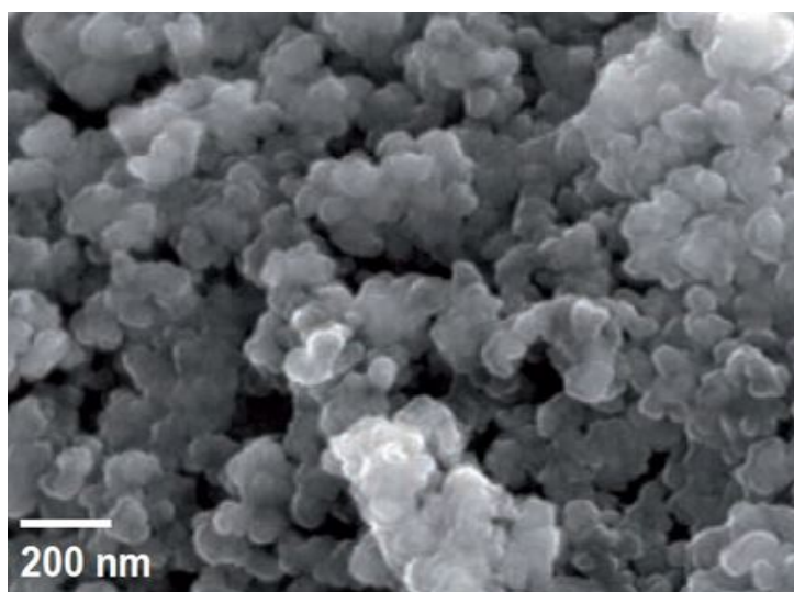
SEM – Ytria Stabilized Zirconia
