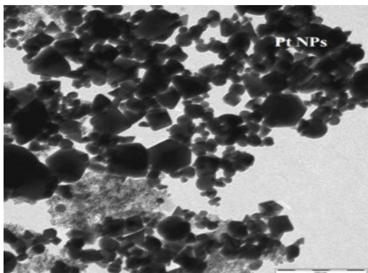
TEM - Pt Nanoparticles
