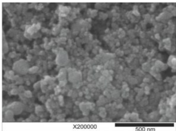
SEM - ZrO 2 Nanoparticles
