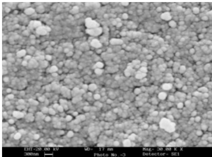
SEM - Zinc Oxide
