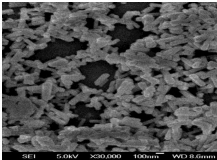
SEM - CdSe Nanorods
