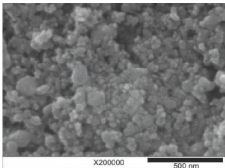
SEM - Zirconium Oxide
