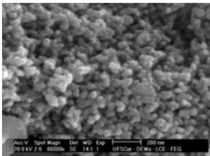
SEM - Indium Tin Oxide
