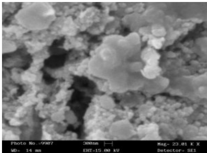
SEM - ATO Nanoparticles
