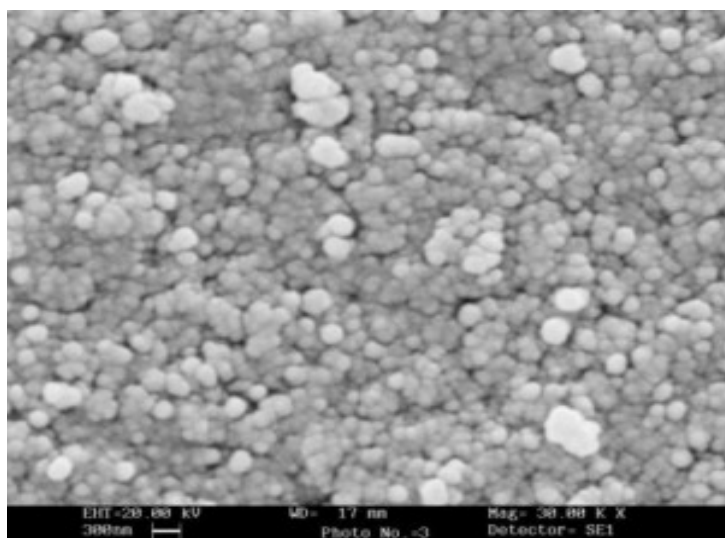
SEM - Zinc Oxide
