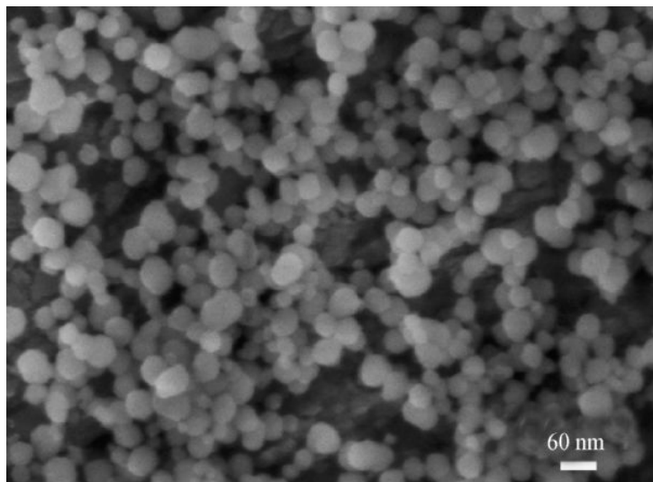
SEM - Ca 2 O 4 Si Nanopowder
