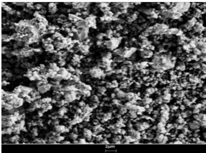
SEM - MoSi 2 Powder
