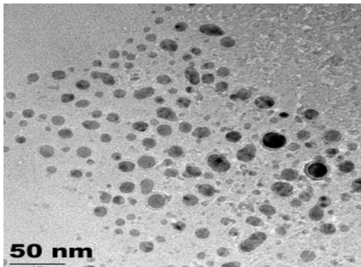
TEM - Indium Arsenide Nanopowder
