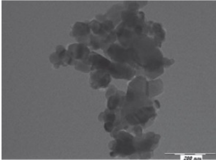
TEM - Gallium Arsenide Powder
