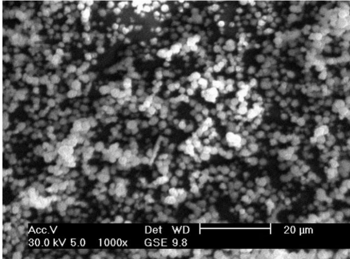
SEM - Zinc Selenide Powder
